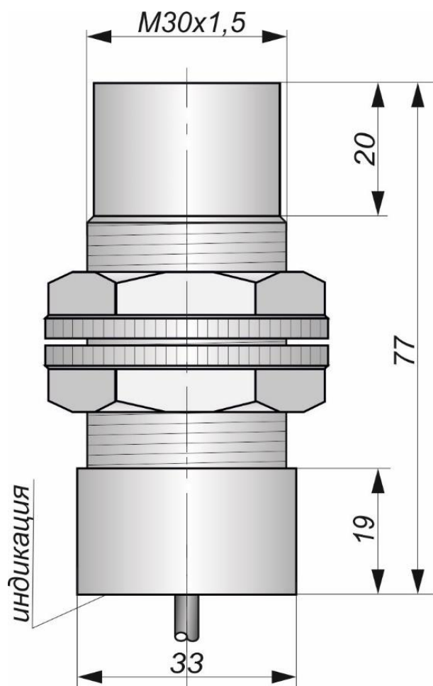
Габаритный чертеж
